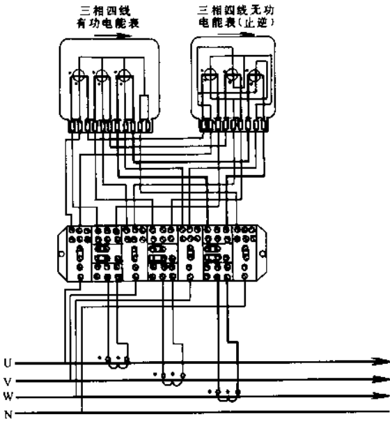
图 A.4 低压计量有功及无功电能电流分相接线方式
