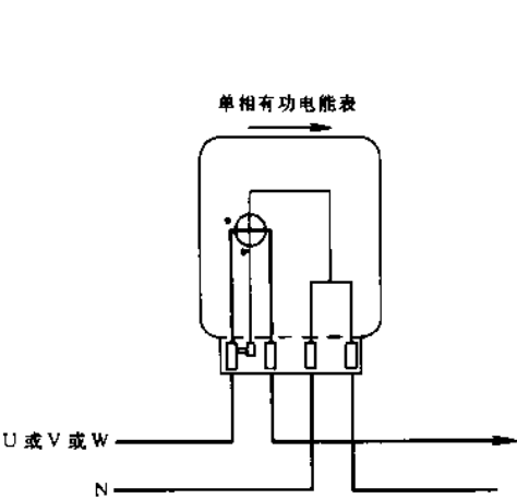
图 A.1 单相计量有功负荷直接接入方式
